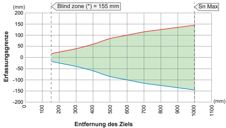
Erfassungskurve mit Rundstab
