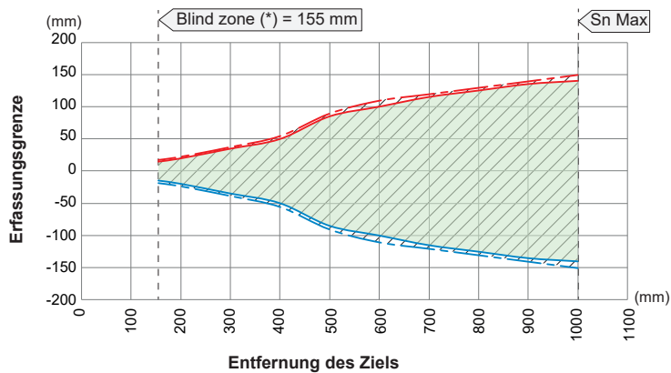
Erfassungskurve mit Rundstab
